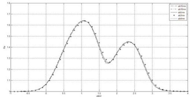
Figura 3. Respuesta del modelo de la Figura 1, para el experimento 1.
