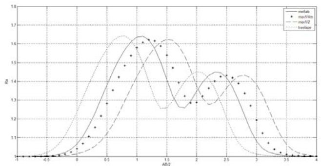
Figura 9. Respuesta del modelo para el experimento 4.
