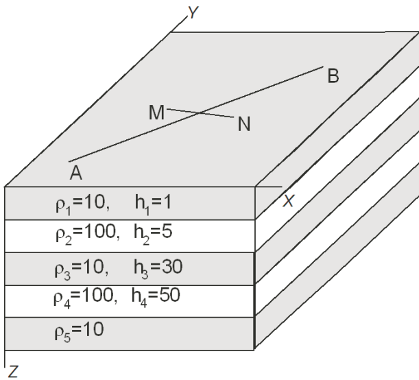
Figura 1. Modelo usado para los cuatro experimentos. La quinta capa, es un semi-espacio homogéneo y no requiere de espesor. Las unidades de la resistividad y espesores son en ohms-metro y en metros, respectivamente.
