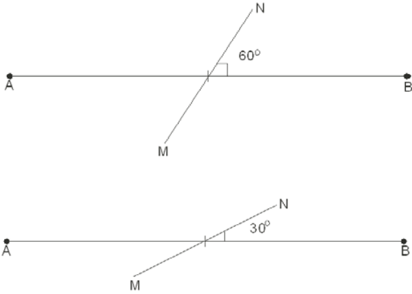
Figura 6. Disposición de los electrodos en el experimento 3. Rotación de M y N
