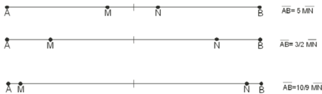
Figura 4. Disposición de los cuatro electrodos para el experimento 2. Los electrodos M y N se van acercando a los electrodos A y B.
