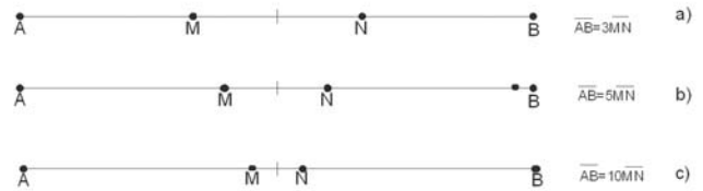
Figura 2. Disposición de los electrodos MN para el experimento 1. Los electrodos M y N se van acercando al punto central.
